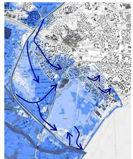
Effacement des digues avec Crue de référence Argens ou crue de référence Reyran
