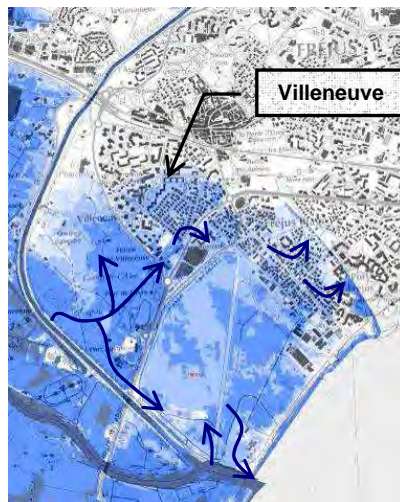
Rupture des digues avec crue de référence de l'Argens & Q10 Reyran
